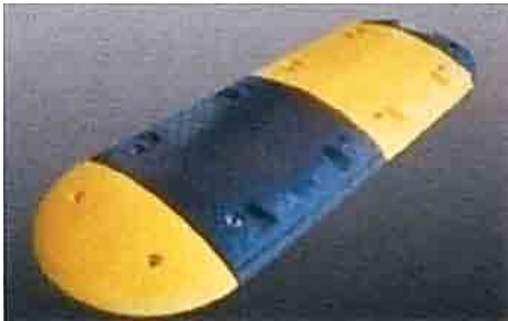
SLC 減速特高大路拱 Size:500 × 430 × 70mm( 中段 ) Size:210 × 430 × 70mm( 端頭 )
