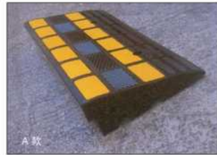
橡膠斜臺 (A) 用途: 樓級, 上平臺, 上門口, 上行人路, 車房門口, 可幫助傷殘人士。 尺寸: 600mm*320mm*100mm
