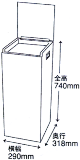
外觀寸法
